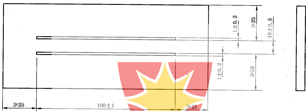
图5 涂导电漆电极的试件
