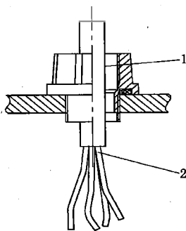
b) 导管引入方式
